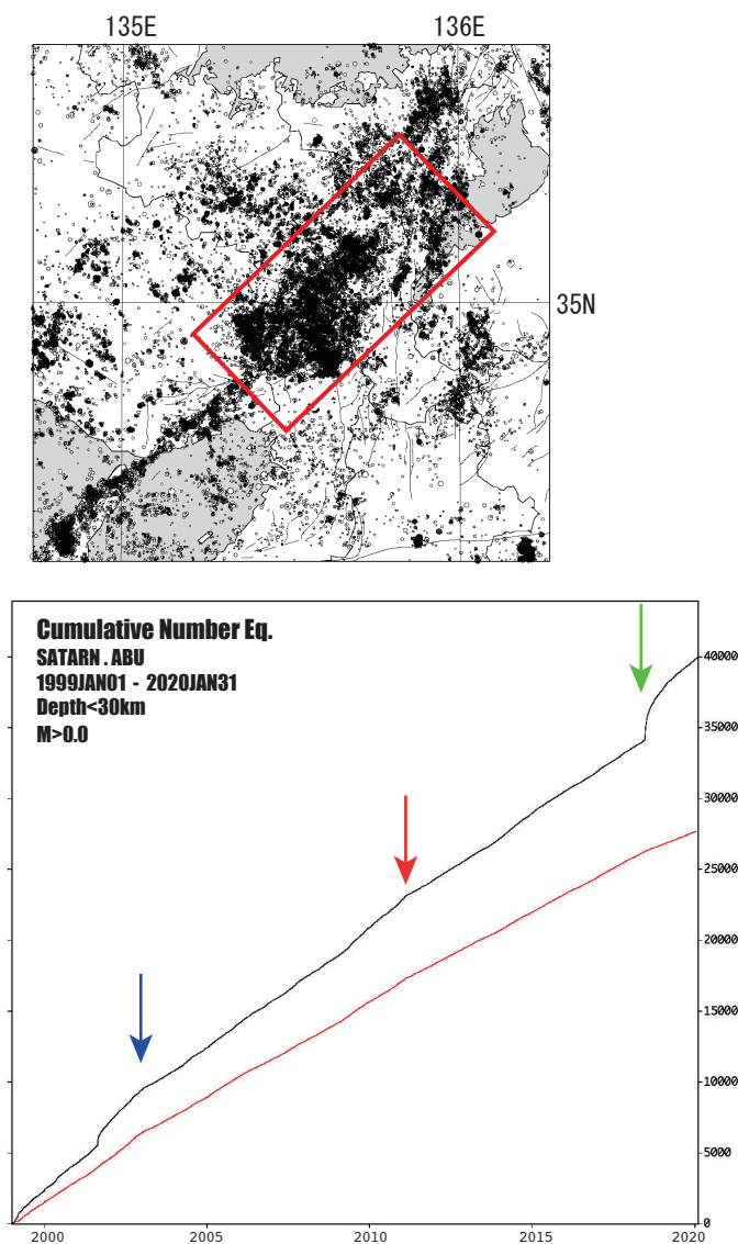
図1：上に示す近畿地方北部の矩形範囲内における積算地震発生数。1999年1月～2020年1月31日。京都大学防災研究所地震予知研究センターによる。
