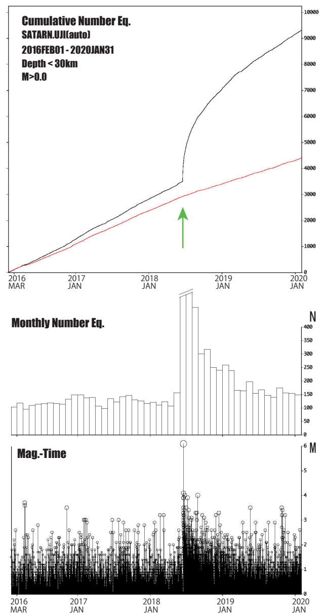
図2：(上) 図1上に示す近畿地方北部の矩形範囲内における積算地震発生数。京都大学防災研究所地震予知研究センターによる。赤線は decluster したカタログによるもの。2016年2月1日～2020年1月31日、30km以浅。(中) 同範囲内での月別地震発生数。(下) 同じく気象庁一元化震源に基づくMT図。
