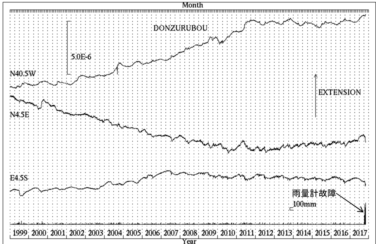
第2図 屯鶴峯観測所における歪変化と日雨量 (1999年1月～2017年10月)
