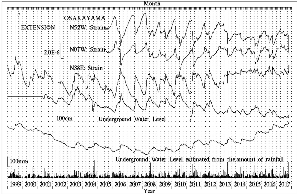
第1図 逢坂山観測所における歪変化、地下水位と日雨量(1999年1月～2017年10月)
