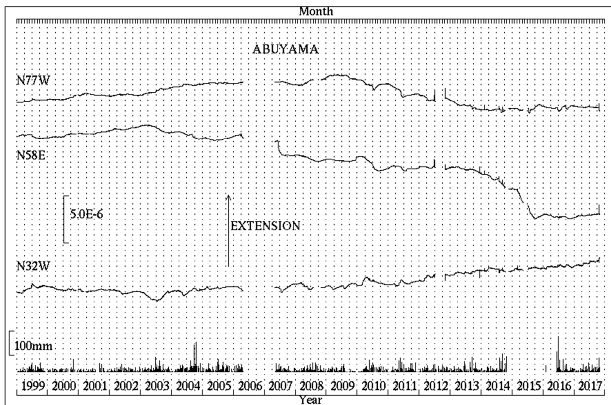
第3図 阿武山観測所における歪変化と日雨量（1999年1月～2017年10月）
