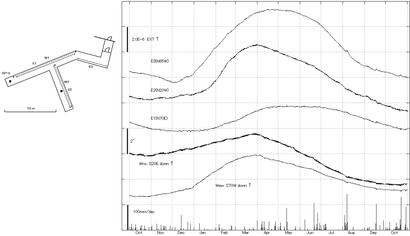
第9図 宿毛観測所における歪・傾斜変化と日雨量(2016年10月～2017年10月)
