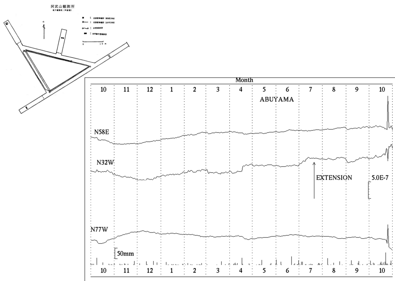
第3図 阿武山観測室における歪変化と日雨量(2016年10月～2017年10月)
