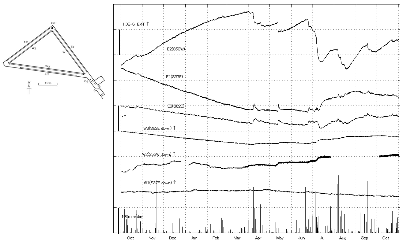
第8図 伊佐観測室における歪・傾斜変化と日雨量(2016年10月～2017年10月)
