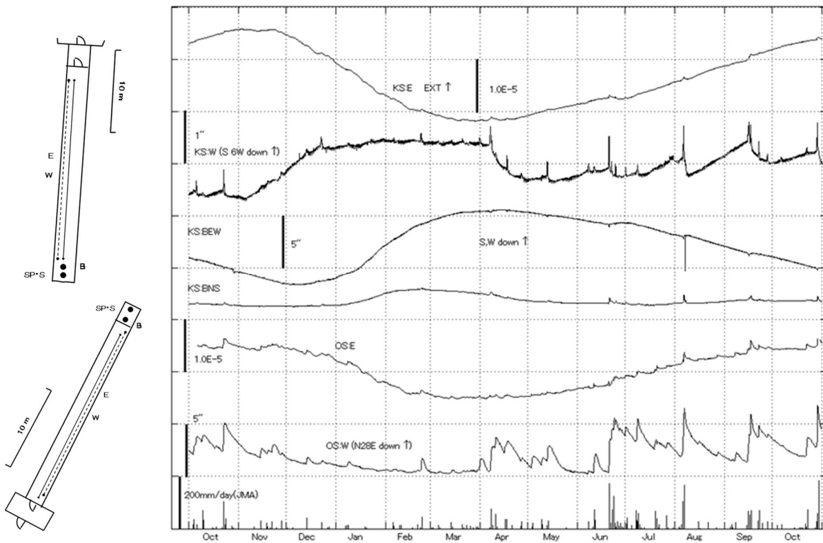
第6図 串間・大隈, 観測室における歪変化と傾斜変化(2016年10月～2017年10月) 雨量はアメダス(鹿児島県田代)の日雨量
