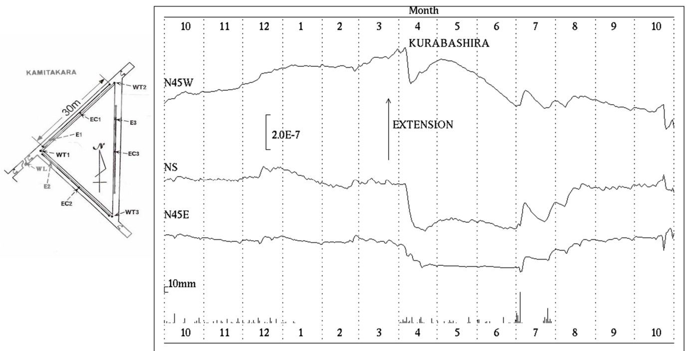
第2図 上宝観測所蔵柱観測室における歪変化と日雨量(2016年10月～2017年10月)
