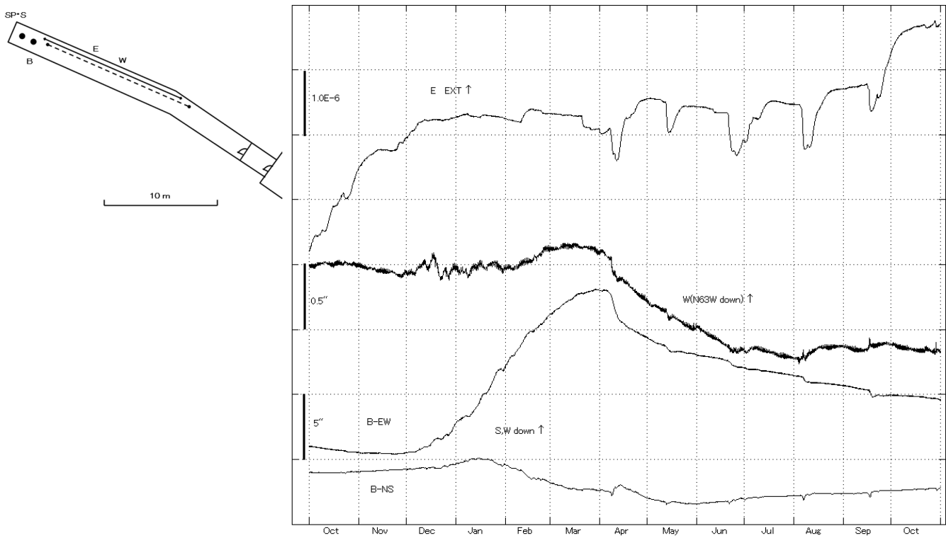
第10図 高城観測室における歪変化と傾斜変化(2016年10月～2017年10月)
