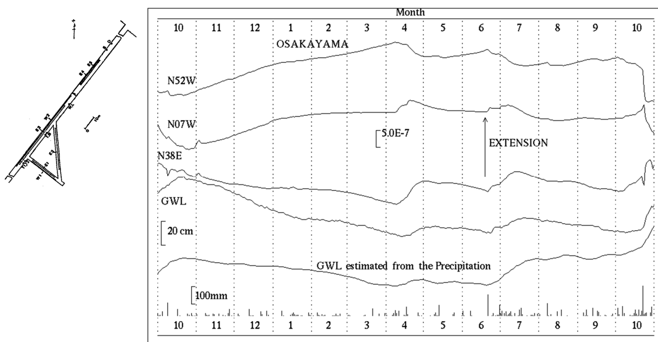
第4図 逢坂山観測室における歪変化と日雨量(2016年10月～2017年10月)
