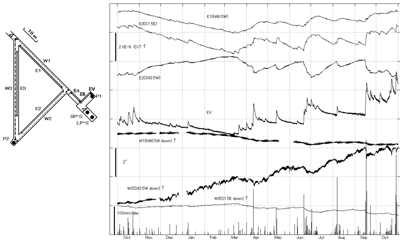
第7図 宮崎観測室における歪・傾斜変化と日雨量(2016年10月～2017年10月)
