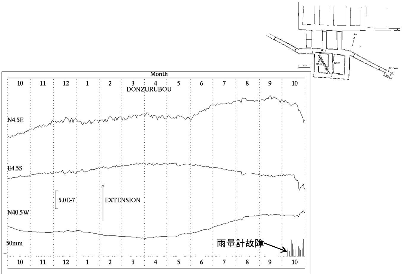
第5図 屯鶴峯観測所における歪変化と日雨量(2016年10月～2017年10月)
