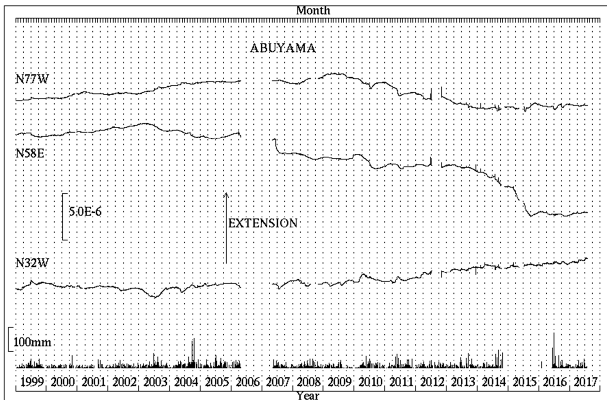
第3図 阿武山観測所における歪変化と日雨量（1999年1月～2017年7月）
