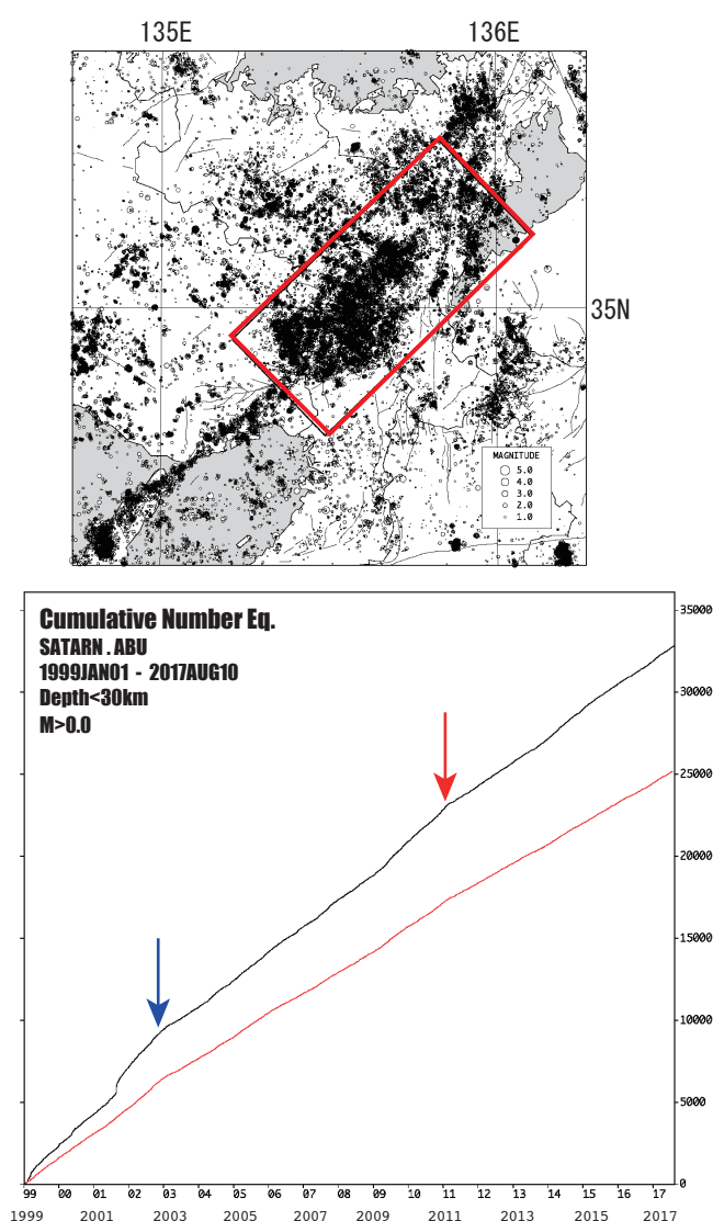
図1：上に示す近畿地方北部の矩形範囲内における積算地震発生数。1999年1月～2017年8月10日。京都大学防災研究所地震予知研究センターによる。
