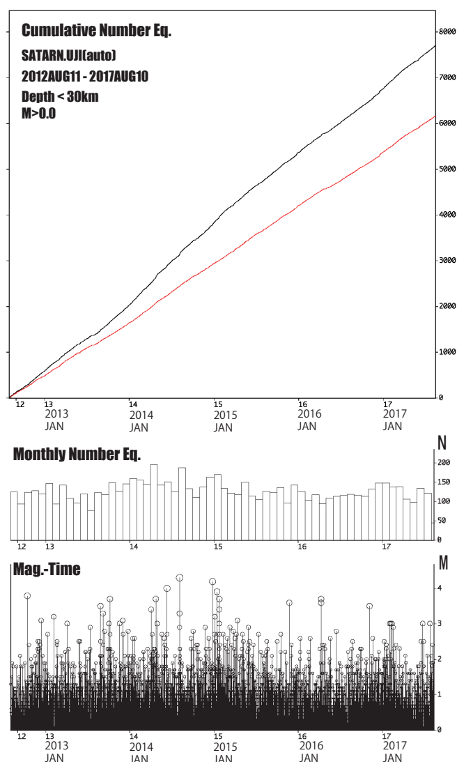
図2：(上) 図1上に示す近畿地方北部の矩形範囲内における積算地震発生数。京都大学防災研究所地震予知研究センターによる。赤線は decluster したカタログによるもの2012年8月11日～2017年8月10日、30km以浅。
