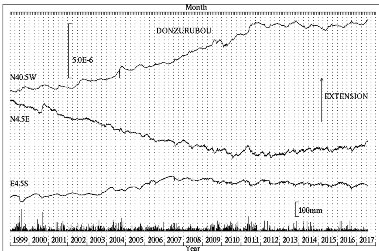
第2図 屯鶴峯観測所における歪変化と日雨量 (1999年1月～2017年7月)
