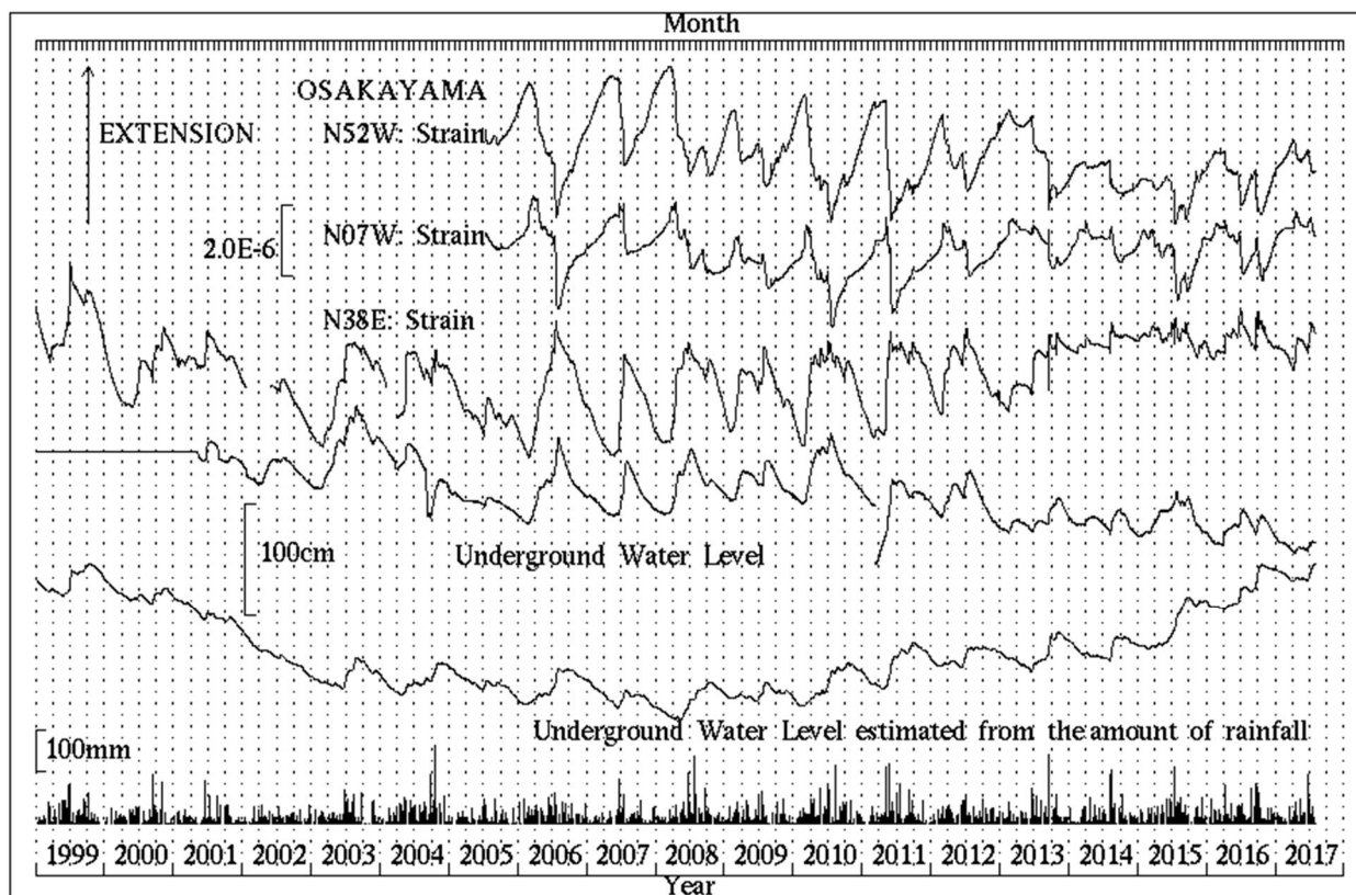
第1図 逢坂山観測所における歪変化、地下水位と日雨量(1999年1月～2017年7月)
