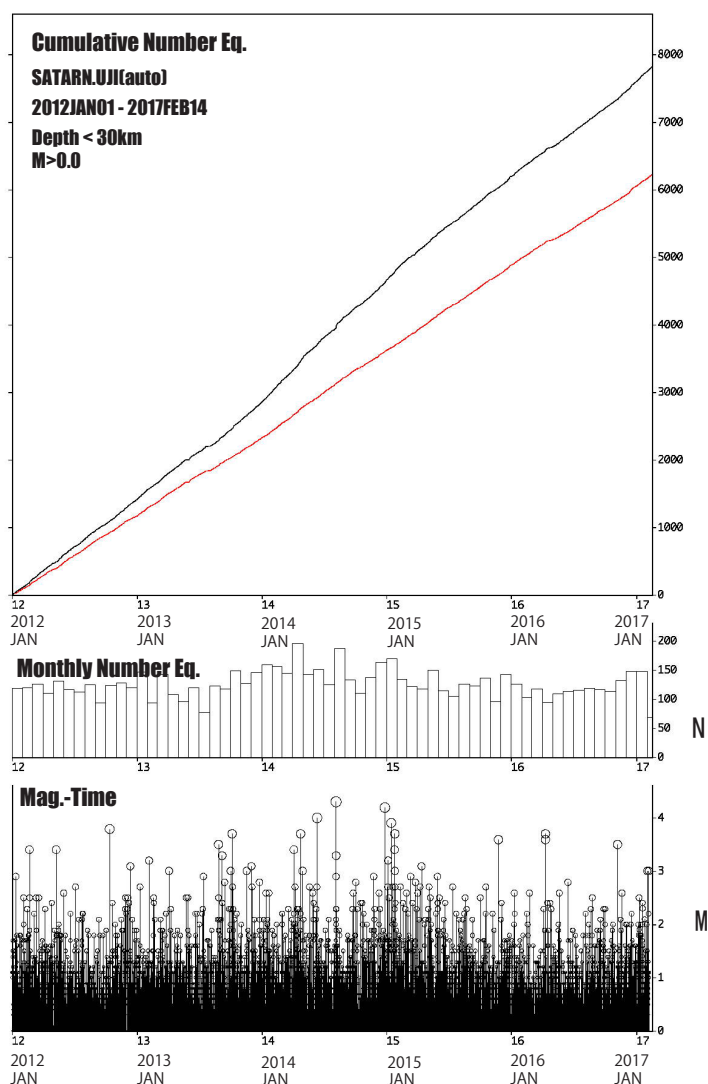
図2：(上) 図1上に示す近畿地方北部の矩形範囲内における積算地震発生数。京都大学防災研究所地震予知研究センターによる。赤線は decluster したカタログによるもの。2012年1月1日～2017年2月14日、30km以浅。
