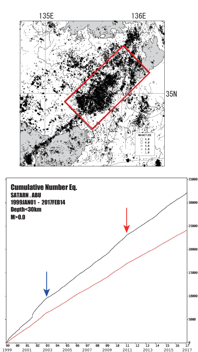
図1：上に示す近畿地方北部の矩形範囲内における積算地震発生数。1999年1月～2017年2月14日。京都大学防災研究所地震予知研究センターによる。
