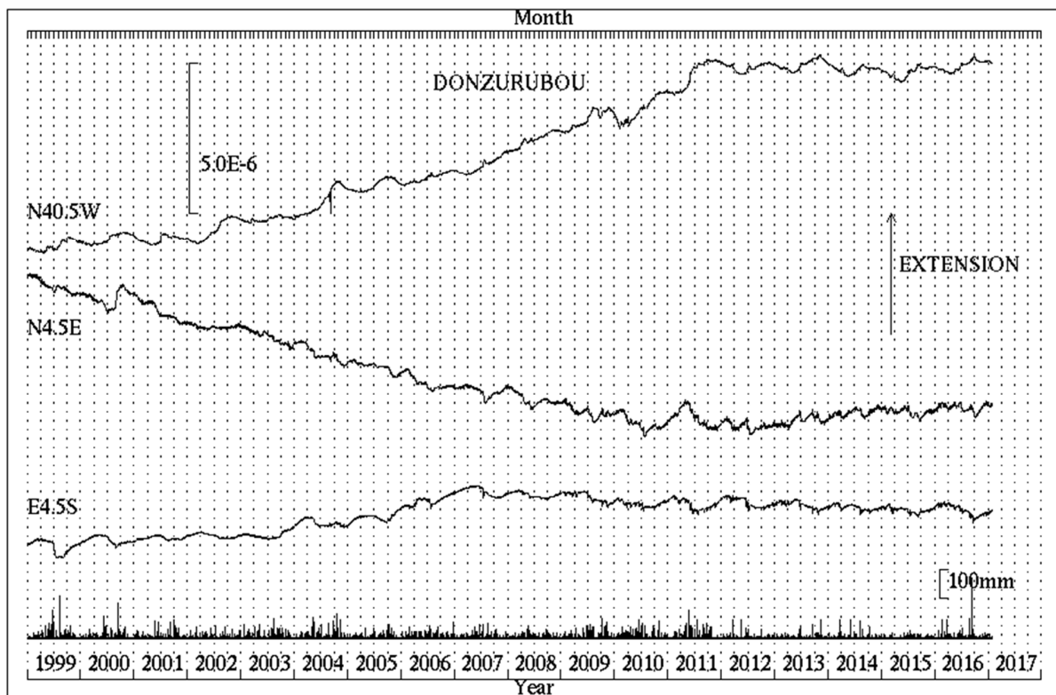
第2図 屯鶴峯観測所における歪変化と日雨量 (1999年1月～2017年1月)
