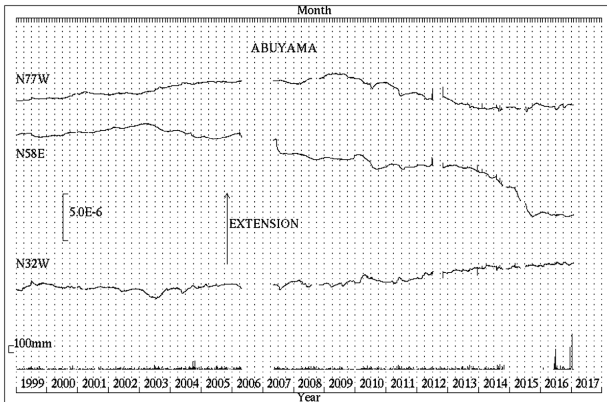
第3図 阿武山観測所における歪変化と日雨量（1999年1月～2017年1月）
