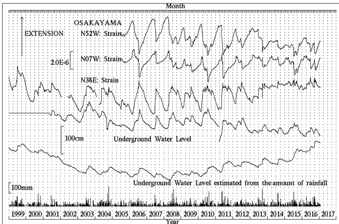
第1図 逢坂山観測所における歪変化、地下水位と日雨量(1999年1月～2017年1月)
