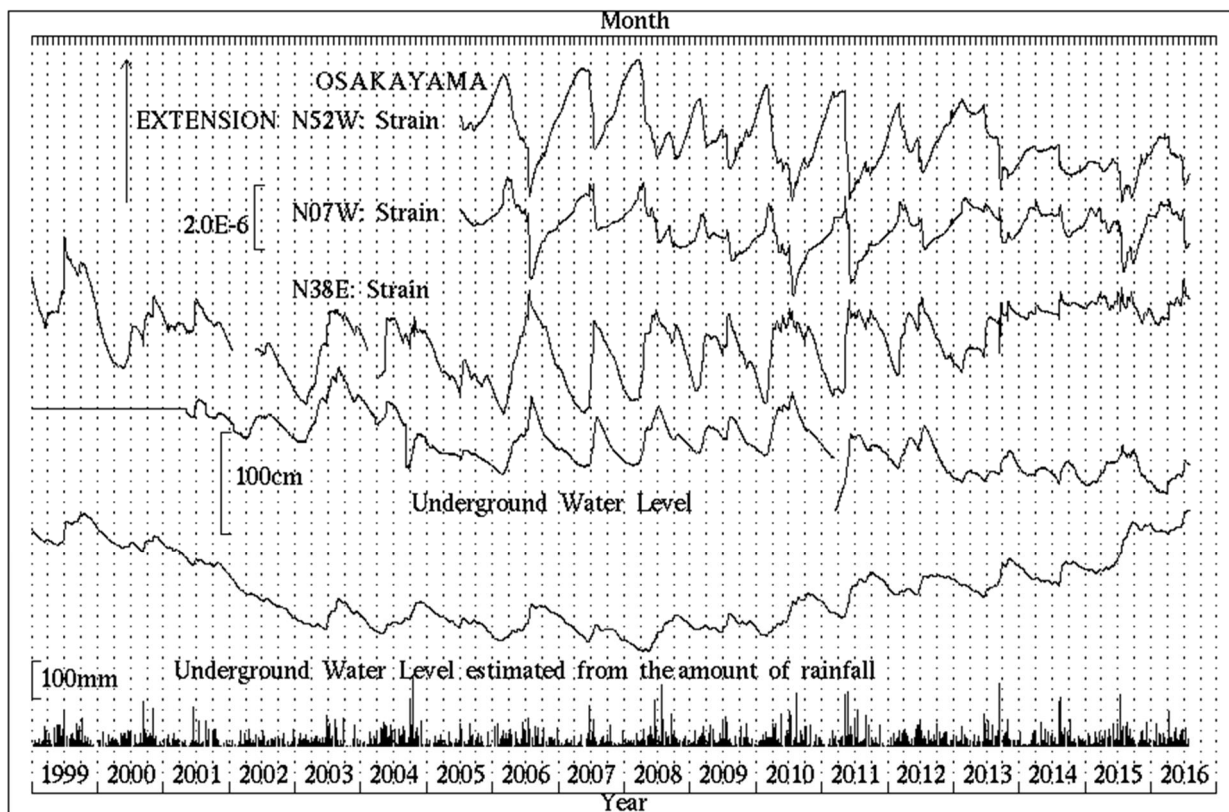
第1図 逢坂山観測所における歪変化、地下水位と日雨量(1999年1月～2016年7月)
