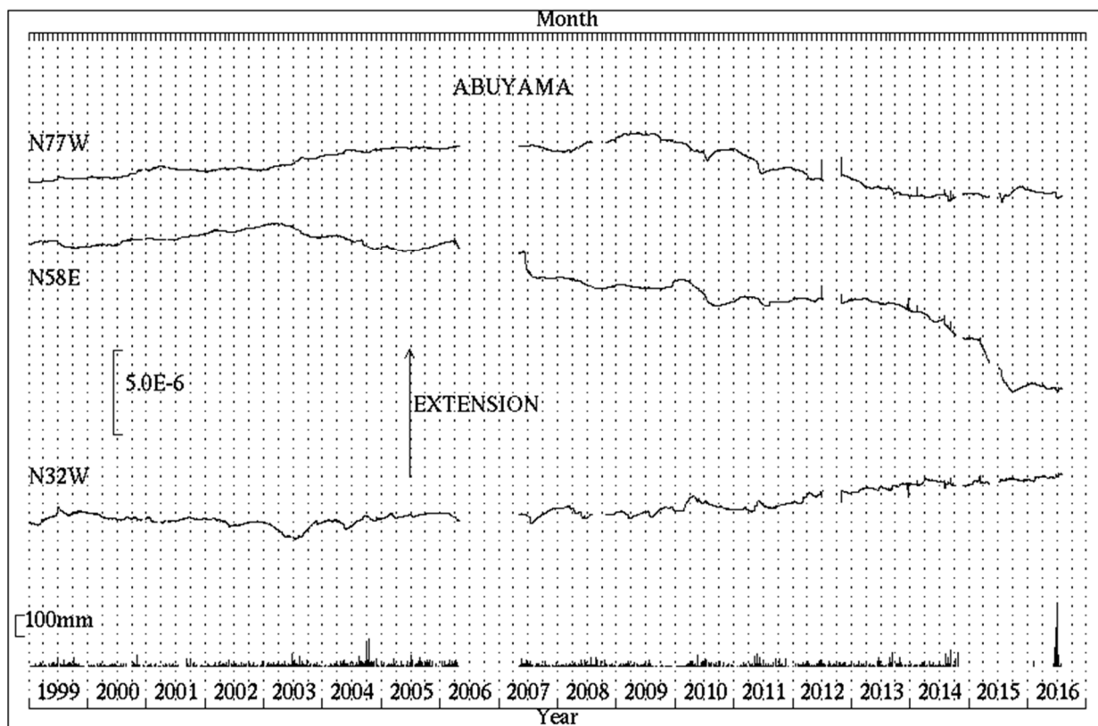
第3図 阿武山観測所における歪変化と日雨量（1999年1月～2016年7月）
