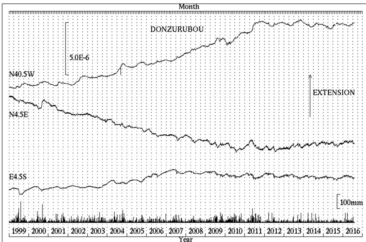
第2図 屯鶴峯観測所における歪変化と日雨量(1999年1月～2016年7月)
