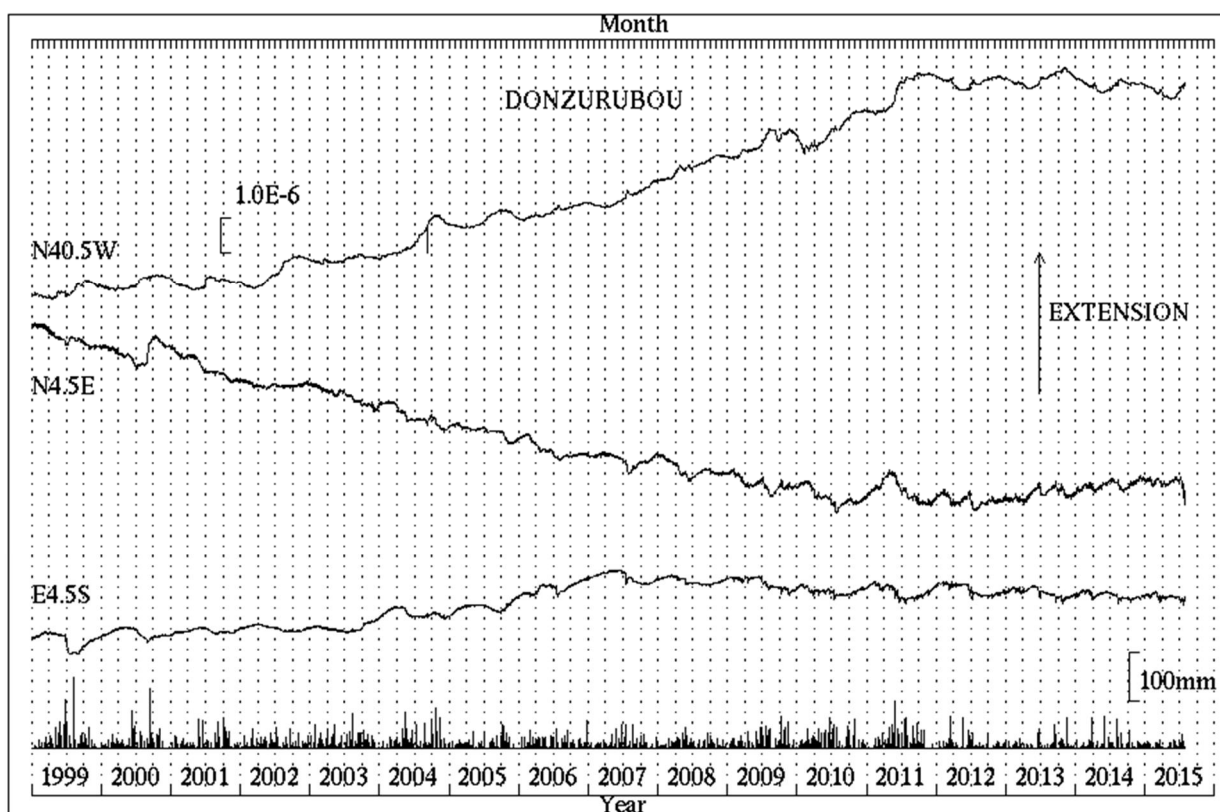
第2図 屯鶴峯観測所における歪変化と日雨量 (1999年1月～2015年7月)
