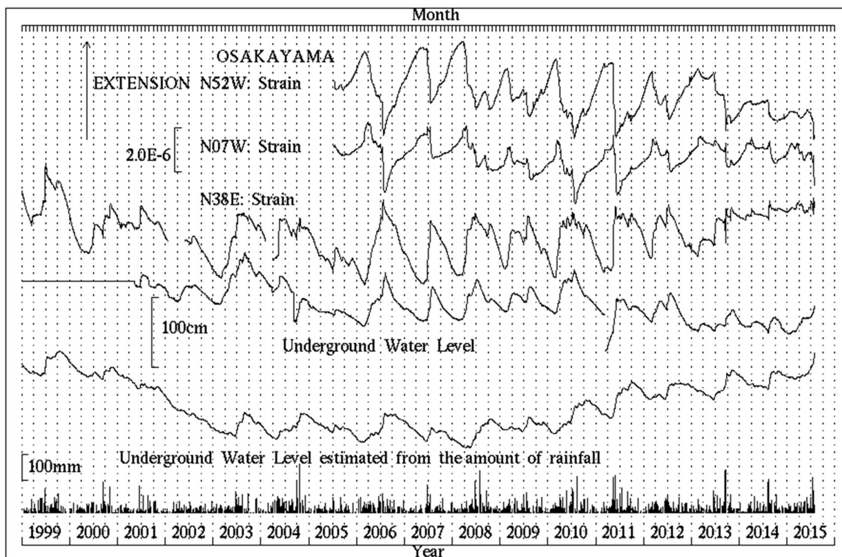
第1図 逢坂山観測所における歪変化、地下水位と日雨量(1999年1月～2015年7月)
