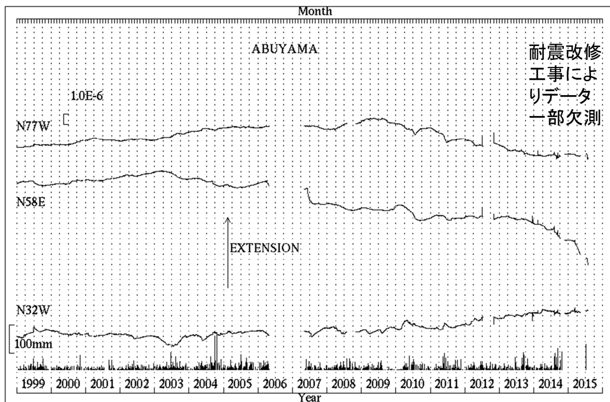
第3図 阿武山観測所における歪変化と日雨量（1999年1月～2015年7月）
