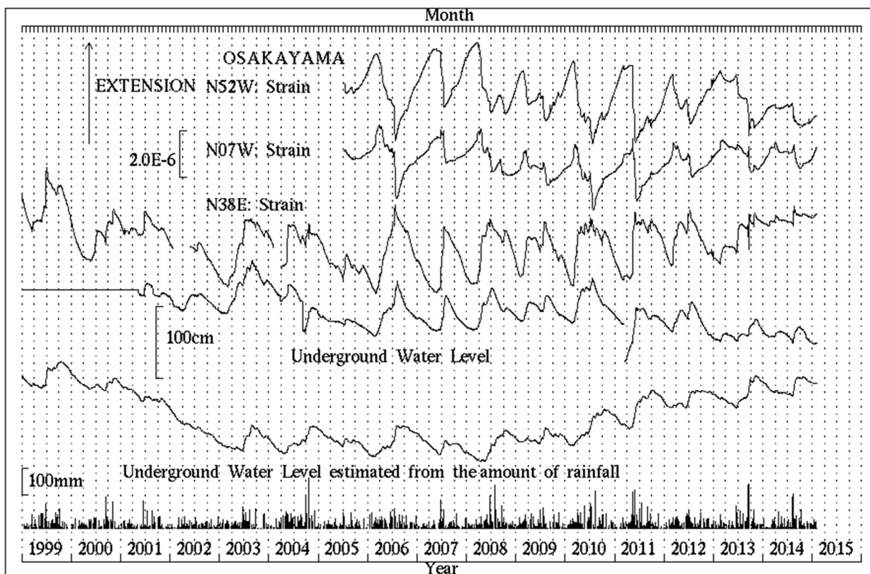
第1図 逢坂山観測所における歪変化、地下水位と日雨量(1999年1月～2015年1月)
