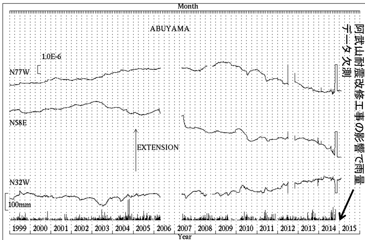
第3図 阿武山観測所における歪変化と日雨量（1999年1月～2015年1月）
