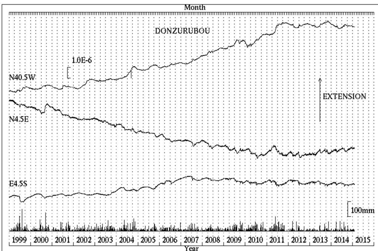
第2図 屯鶴峯観測所における歪変化と日雨量 (1999年1月～2015年1月)
