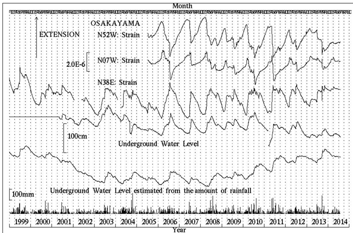
第1図 逢坂山観測所における歪変化、地下水位と日雨量（1999年1月～2014年7月）
