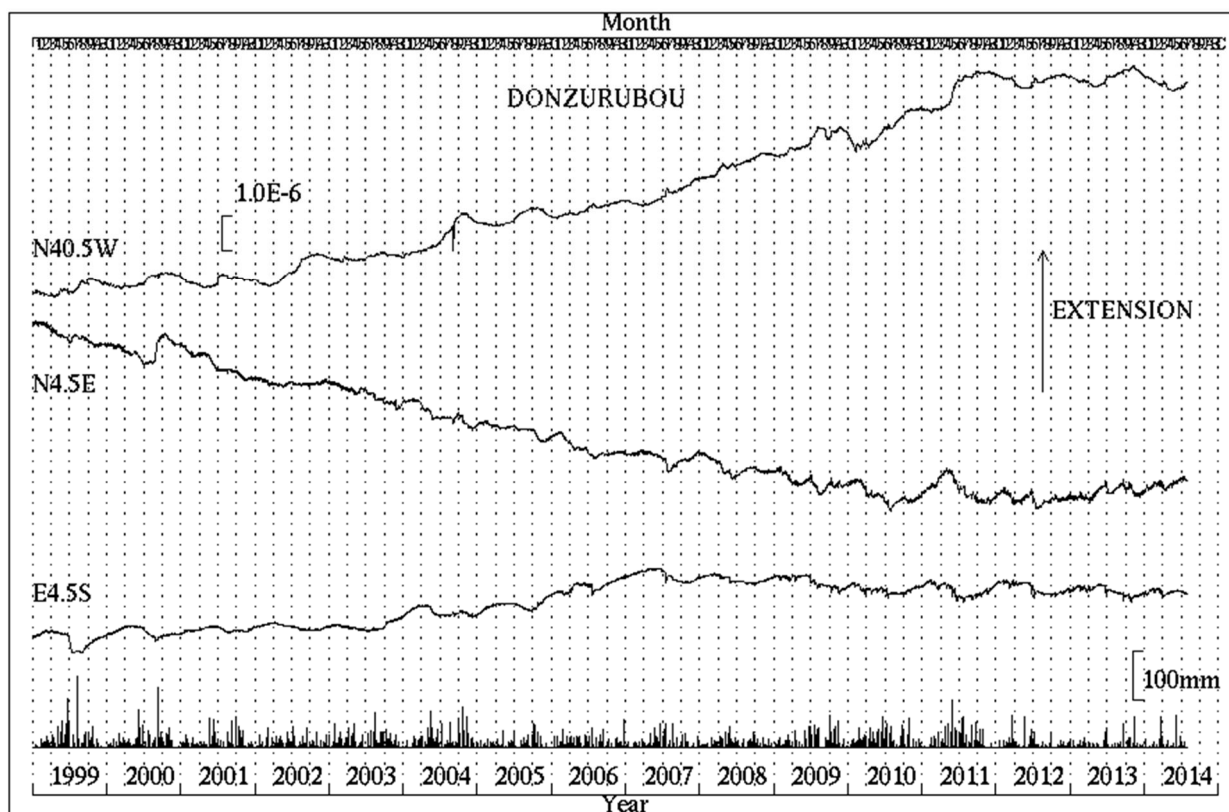
第2図 屯鶴峯観測所における歪変化と日雨量（1999年1月～2014年7月）
