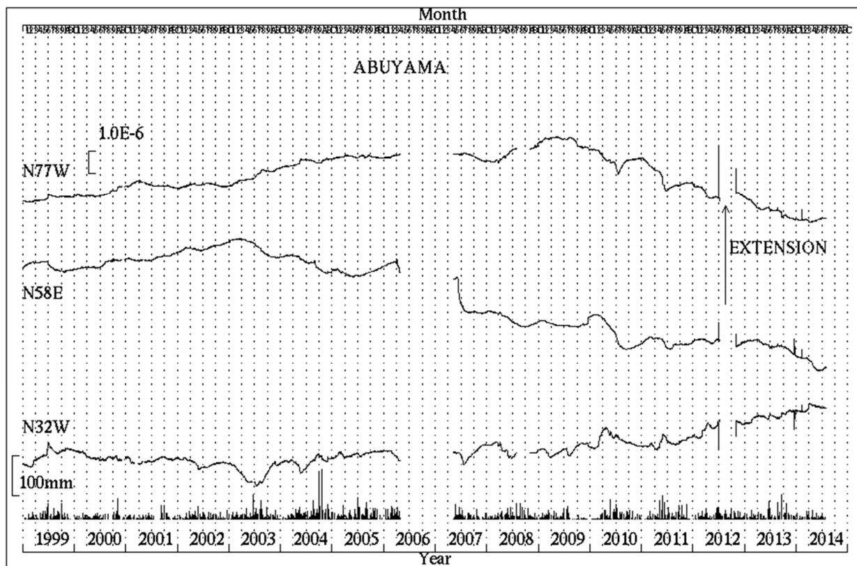
第3図 阿武山観測所における歪変化と日雨量（1999年1月～2014年7月）
