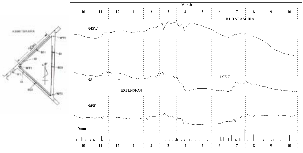
第2図 上宝観測所蔵柱観測室における歪変化と日雨量(2011年10月～2012年10月)
