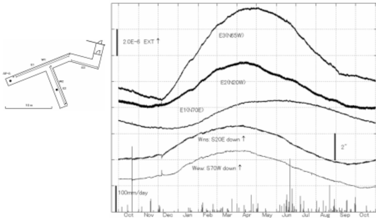
第9図 宿毛観測所における歪・傾斜変化と日雨量(2011年10月～2012年10月)
