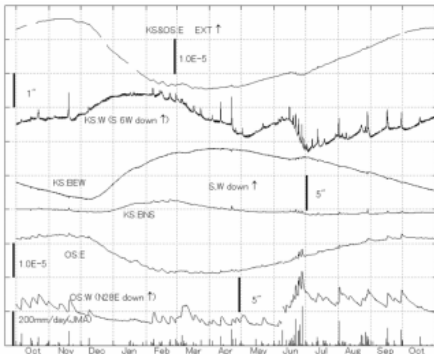
第6図 串間・大隈, 観測室における歪変化と傾斜変化(2011年10月～2012年10月) 雨量はアメダス(鹿児島県田代)の日雨量
