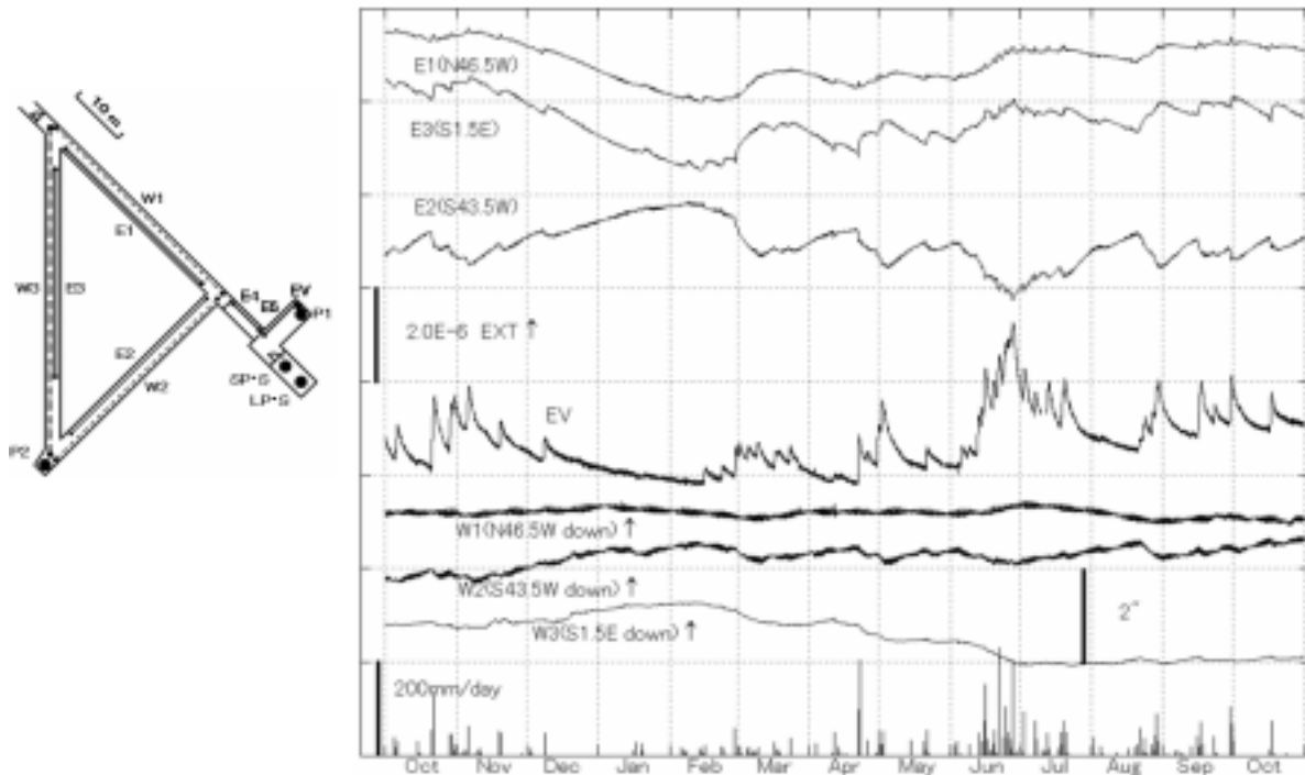
第7図 宮崎観測室における歪・傾斜変化と日雨量(2011年10月～2012年10月)
