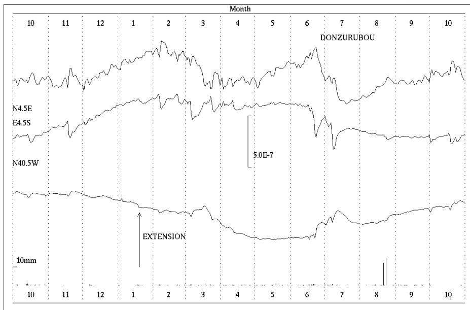
第5図 屯鶴峯観測所における歪変化と日雨量(2011年10月～2012年10月)
