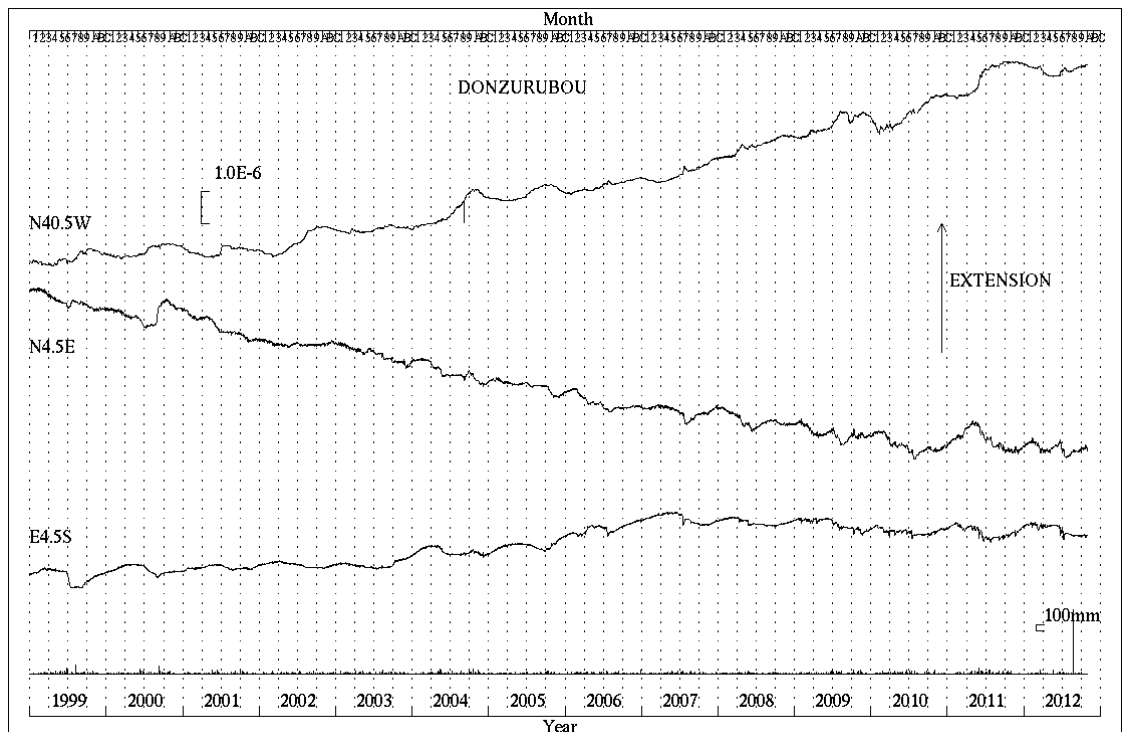
第2図 屯鶴峯観測所における歪変化と日雨量 (1999年1月～2012年10月)
