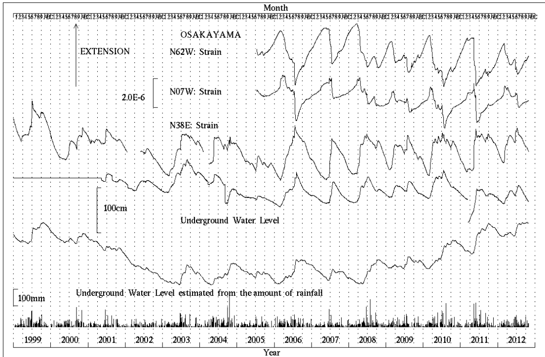
第1図 逢坂山観測所における歪変化、地下水位と日雨量(1999年1月～2012年10月)
