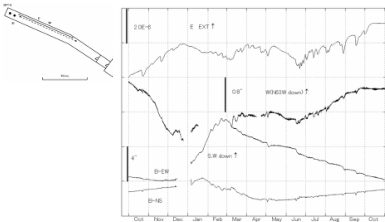
第10図 高城観測室における歪変化と傾斜変化(2011年10月～2012年10月)
