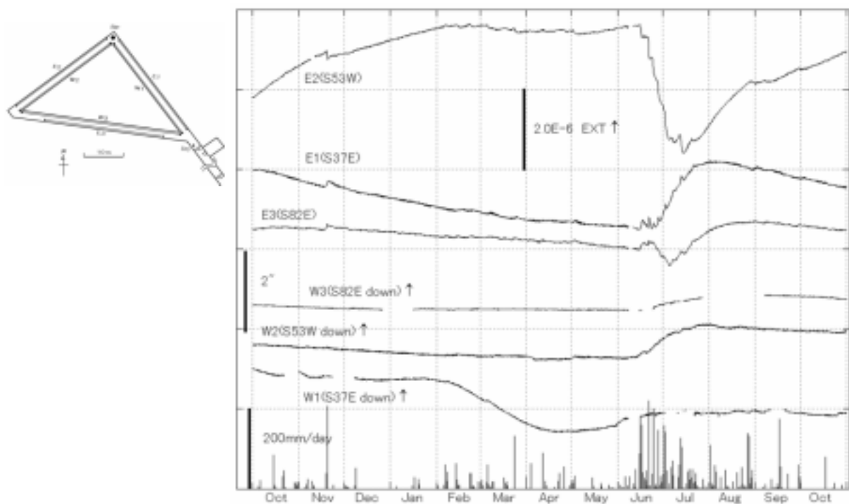
第8図 伊佐観測室における歪・傾斜変化と日雨量(2011年10月～2012年10月)
