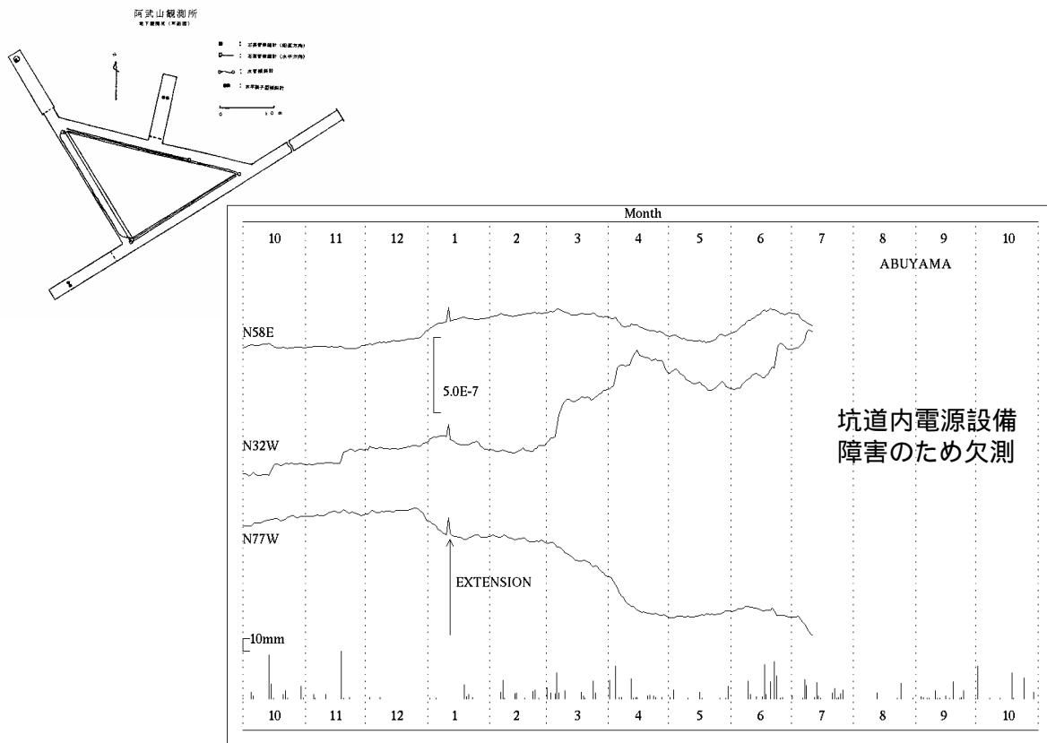
第3図 阿武山観測室における歪変化と日雨量(2011年10月～2012年10月)
