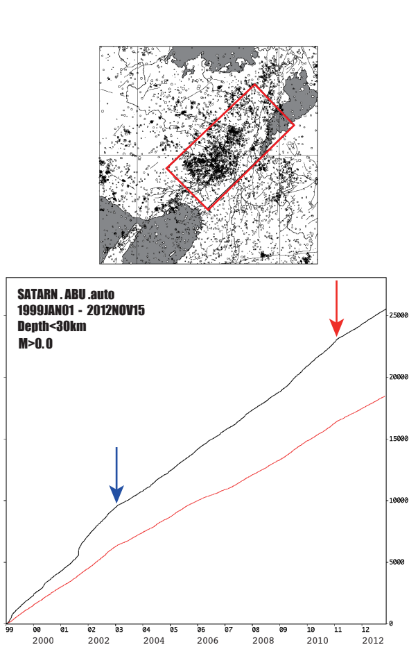
図1：上に示す近畿地方北部の矩形範囲内における積算地震発生数。京都大学防災研究所地震予知研究センターによる。 1999年1月1日～2012年11月15日、30km以浅。 赤矢印は東北地方太平洋沖地震発生時点を示す。 青矢印は丹波山地の静穏化が始まった2003年初頭の時期を示す。赤線は decluster したカタログによる積算発生数。
