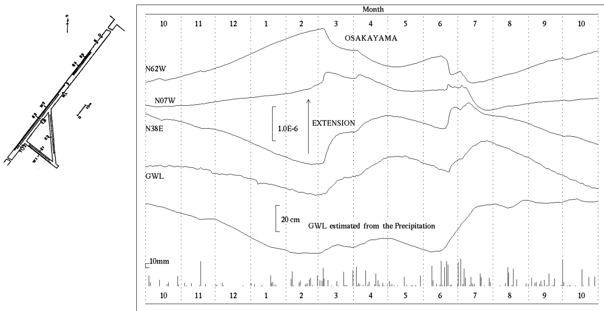
第4図 逢坂山観測室における歪変化と日雨量(2011年10月～2012年10月)
