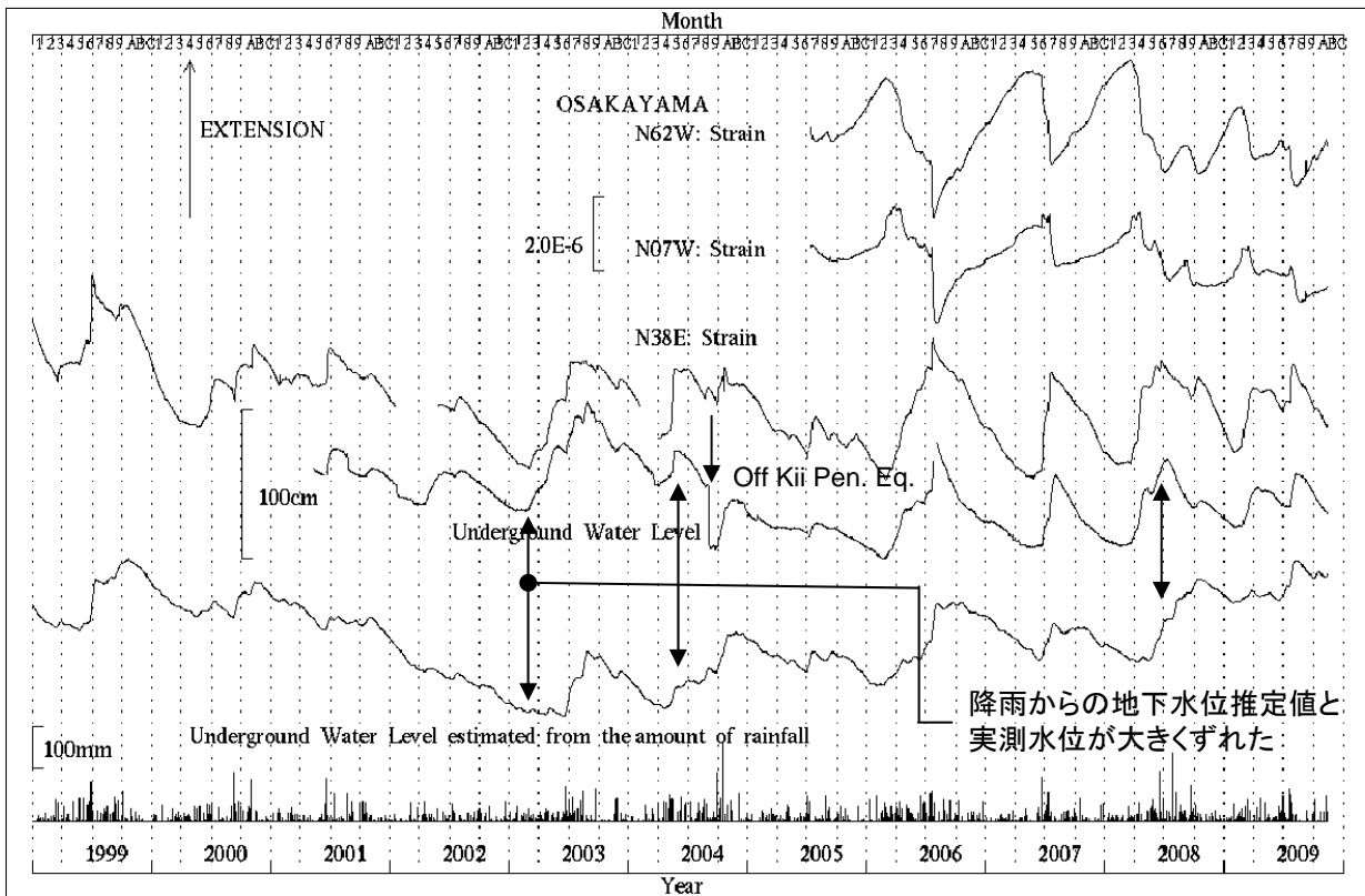
第2図 逢坂山観測所における歪変化、地下水位と日雨量（1999年1月～2009年11月）
