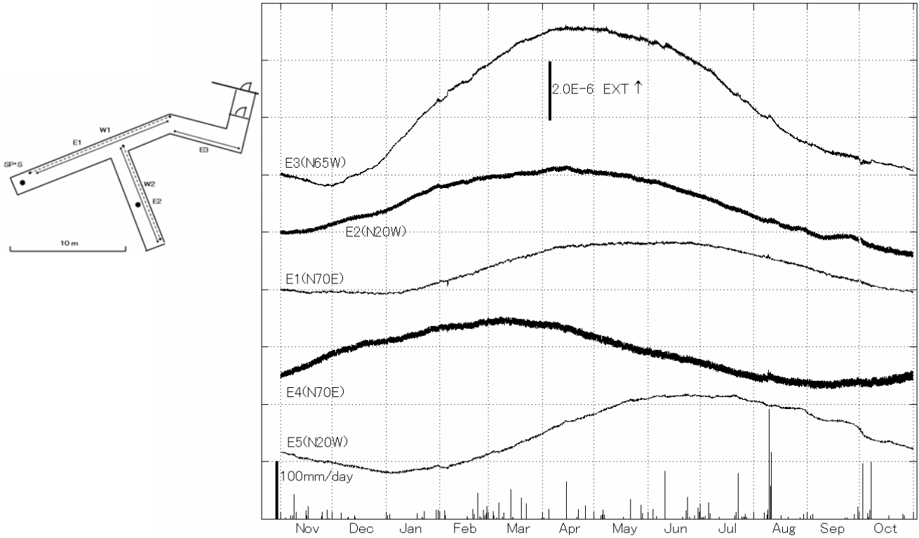
第9図 宿毛観測所における歪変化と日雨量 (2008年11月～2009年10月)
