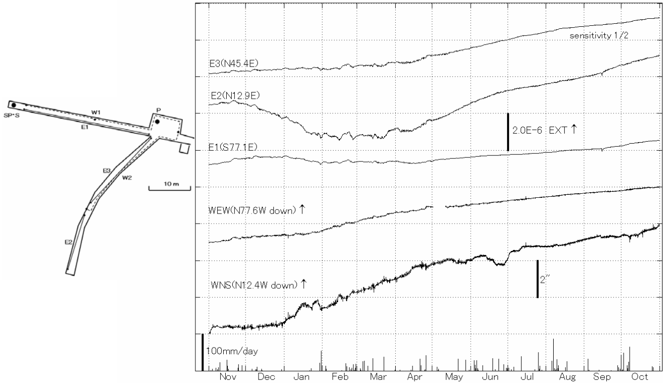
第10図 槇峰観測室における歪・傾斜変化と日雨量 (2008年11月～2009年10月)
