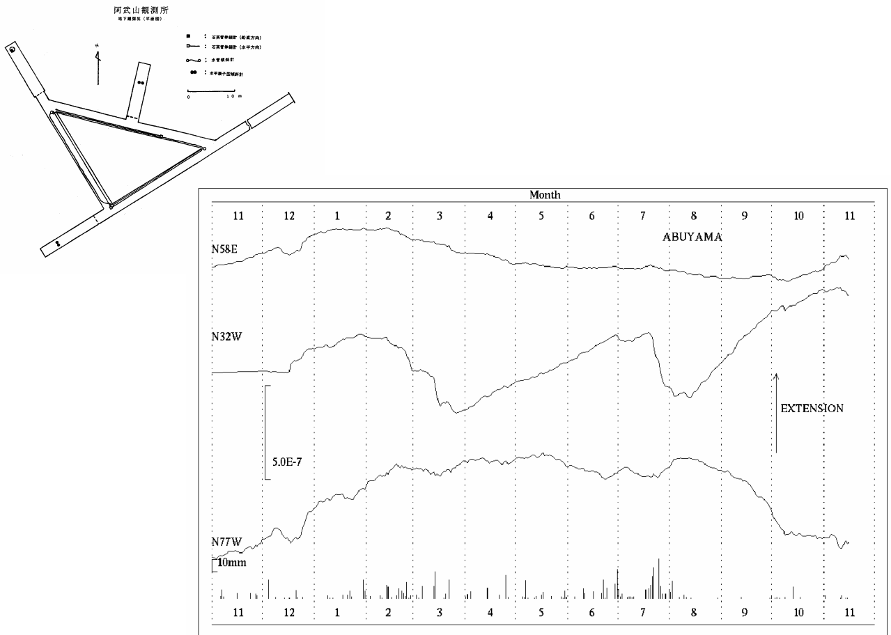
第3図 阿武山観測室における歪変化と日雨量(2008年11月～2009年11月)
