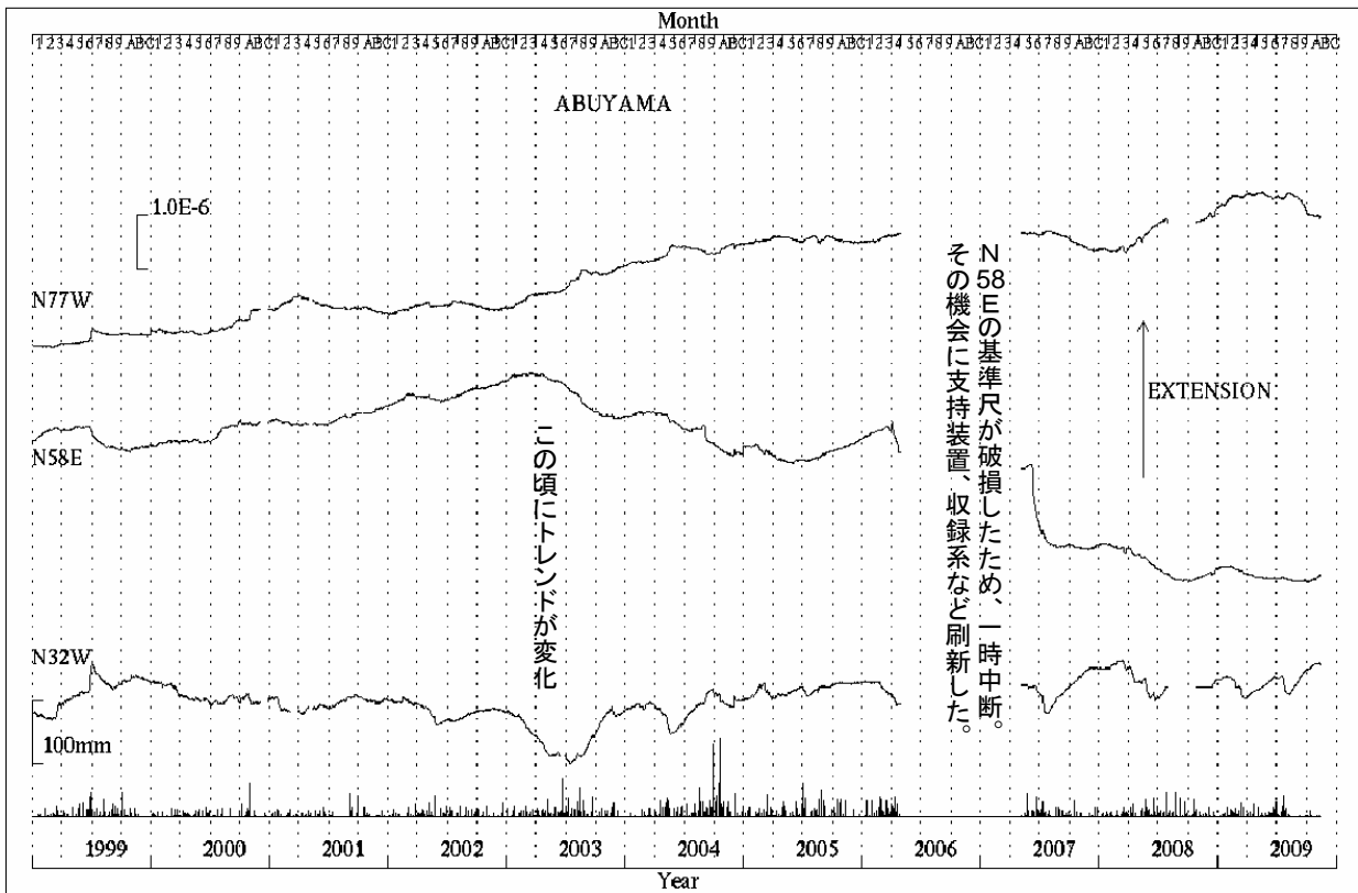
第4図 阿武山観測所における歪変化と日雨量（1999年1月～2009年11月）
