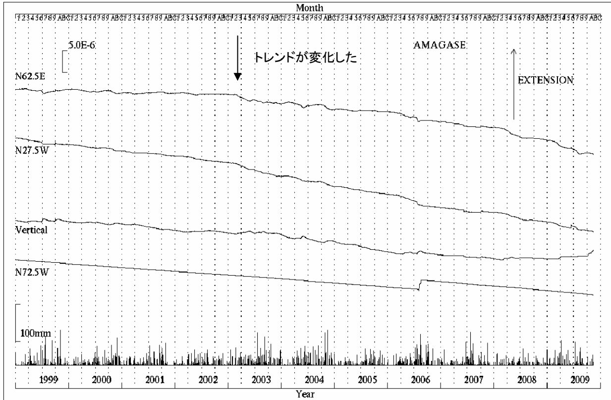
第1図 天ヶ瀬観測室における歪変化と日雨量（1999年1月～2009年11月）
