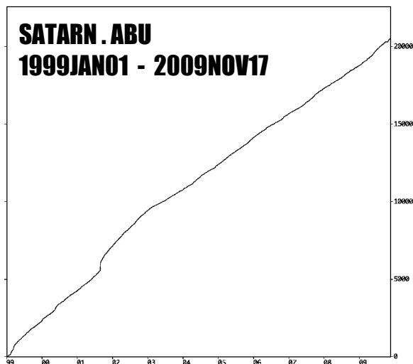
図2：1999年～2009年11月17日、図1の矩形内の積算発生数。
