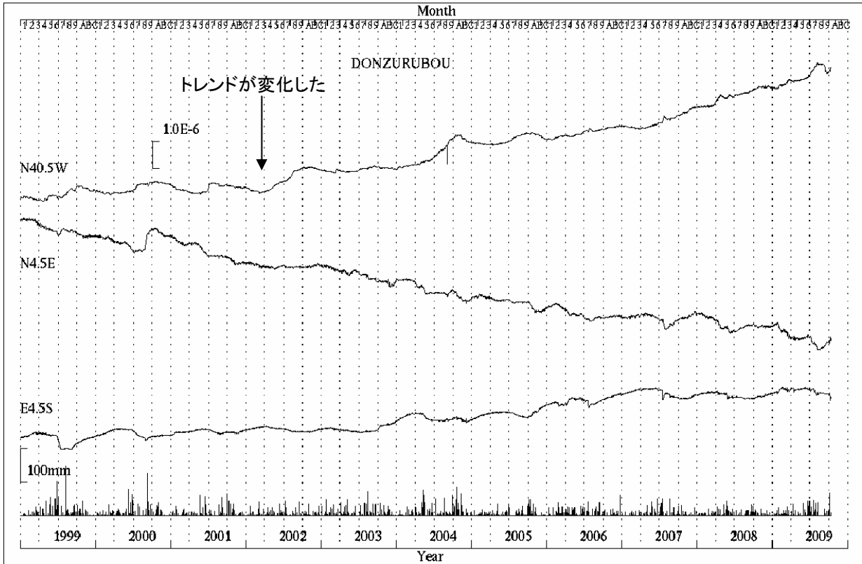
第3図 屯鶴峯観測所における歪変化と日雨量（1999年1月～2009年10月）
