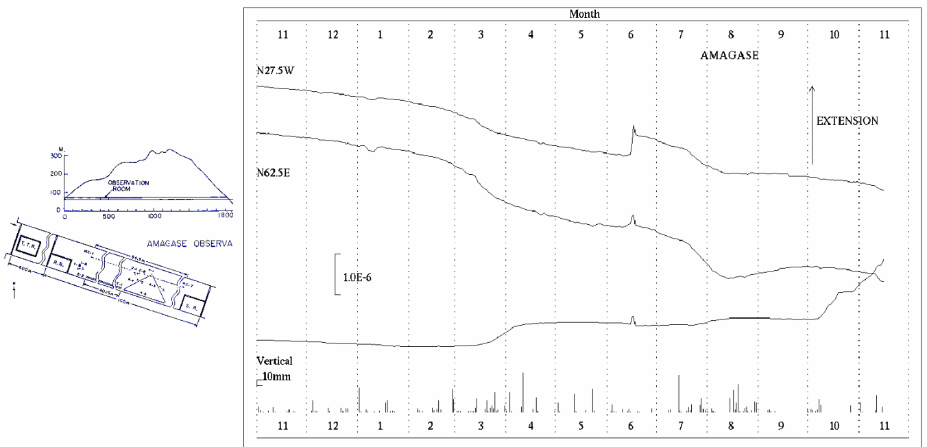
第4図 天ヶ瀬観測室における歪変化と日雨量(2008年11月～2009年11月)
