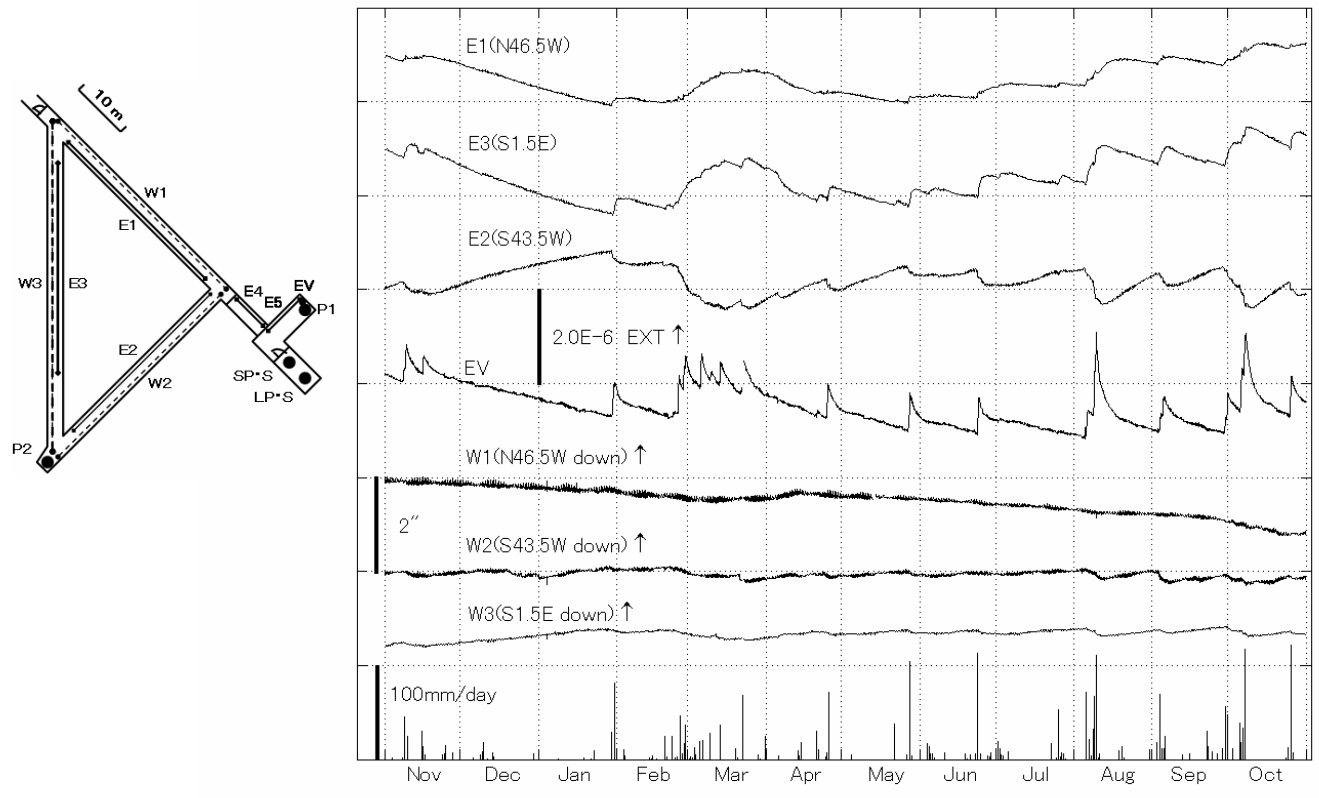
第7図 宮崎観測所における歪・傾斜変化と日雨量(2008年11月～2009年10月)
