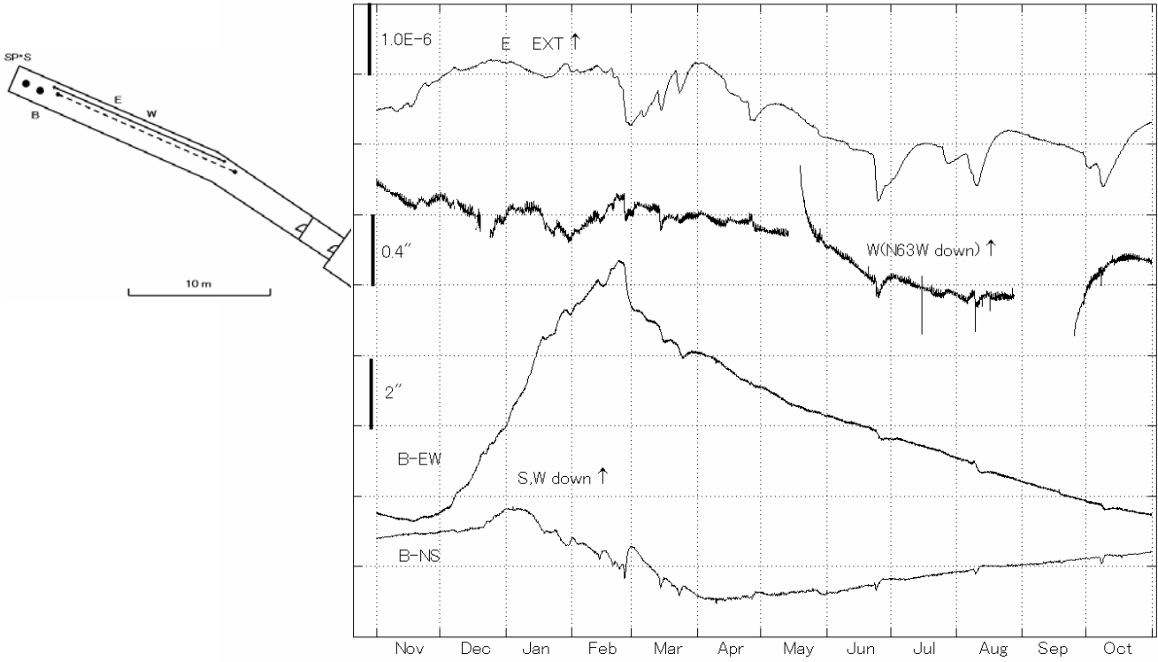
第11図 高城観測室における歪変化と傾斜変化(2008年11月～2009年10月)
