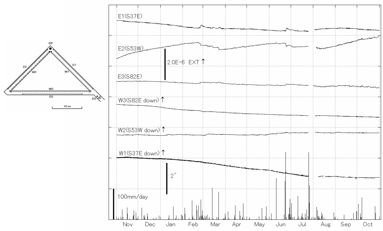
第8図 伊佐観測室における歪・傾斜変化と日雨量(2008年11月～2009年10月)
