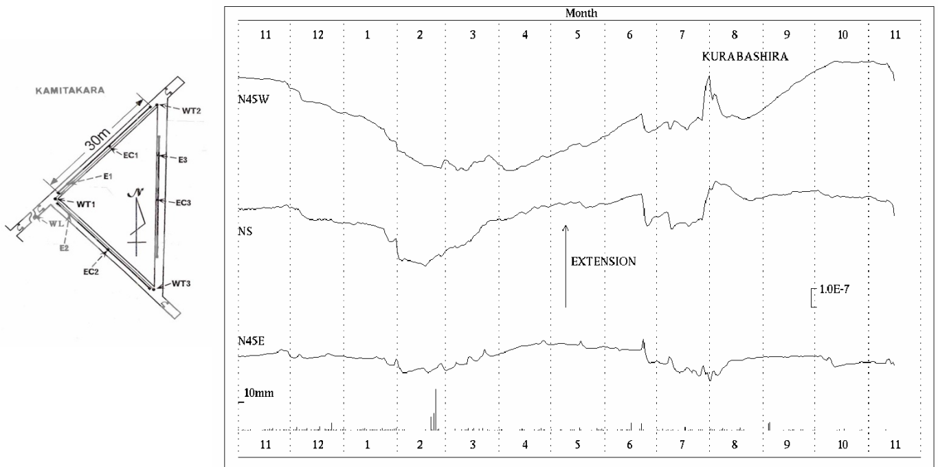
第2図 上宝観測所蔵柱観測室における歪変化と日雨量(2008年11月～2009年11月)
