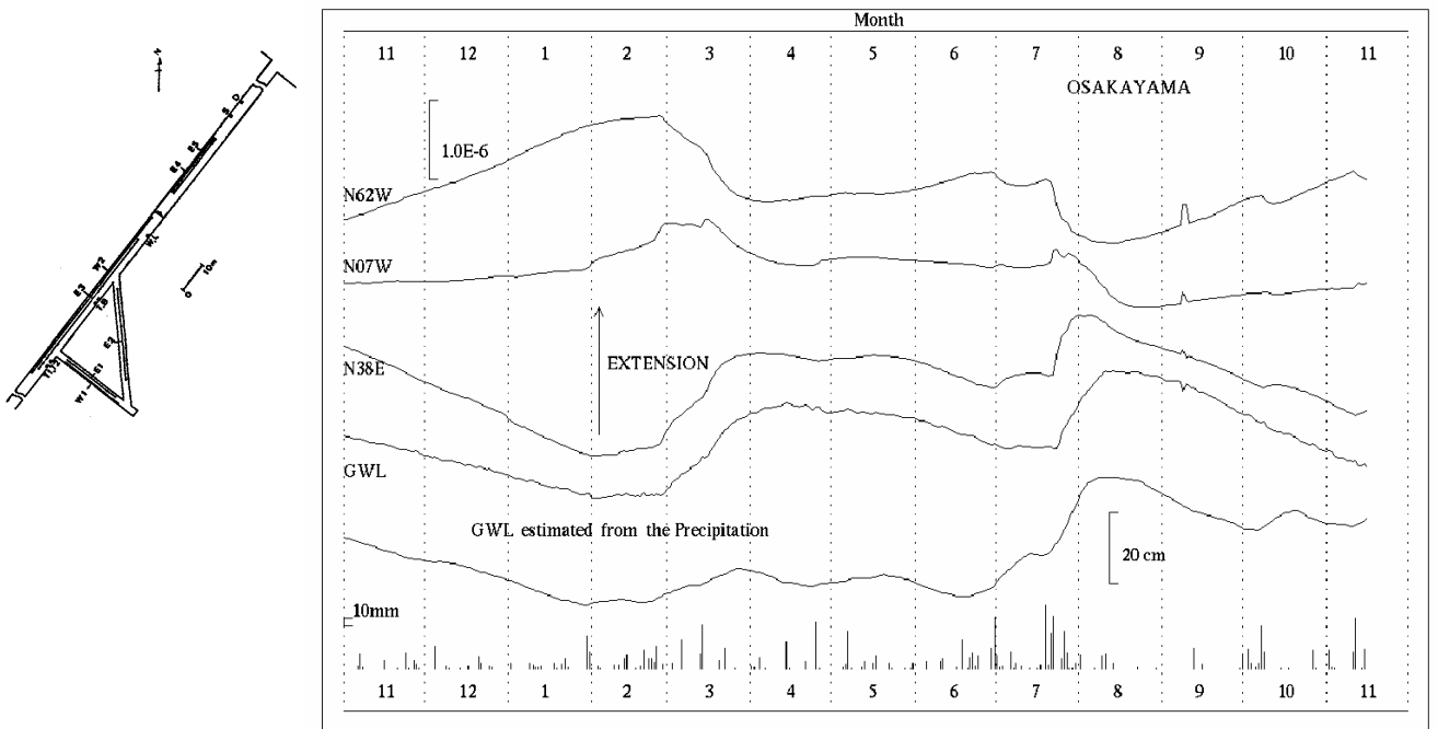
第6図 逢坂山観測所における歪変化、地下水位と日雨量(2008年11月～2009年11月)
