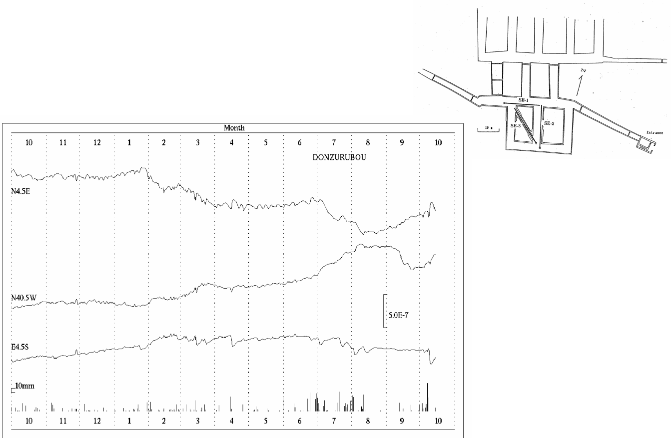
第5図 屯鶴峯観測所における歪変化と日雨量(2008年10月～2009年10月)
