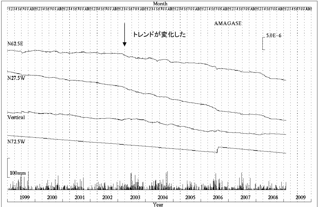
第1図 天ヶ瀬観測室における歪変化と日雨量（1999年1月～2009年2月）
