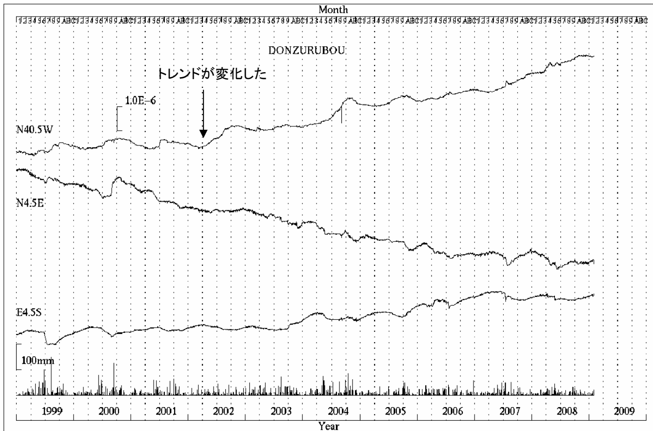
第3図 屯鶴峯観測所における歪変化と日雨量（1999年1月～2009年2月）
