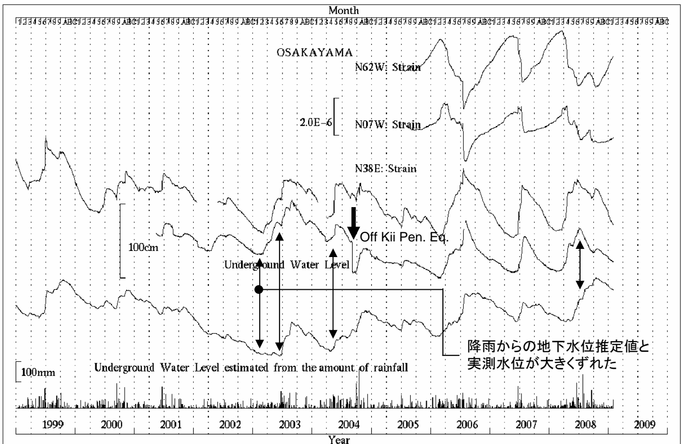
第2図 逢坂山観測所における歪変化、地下水位と日雨量（1999年1月～2009年2月）
