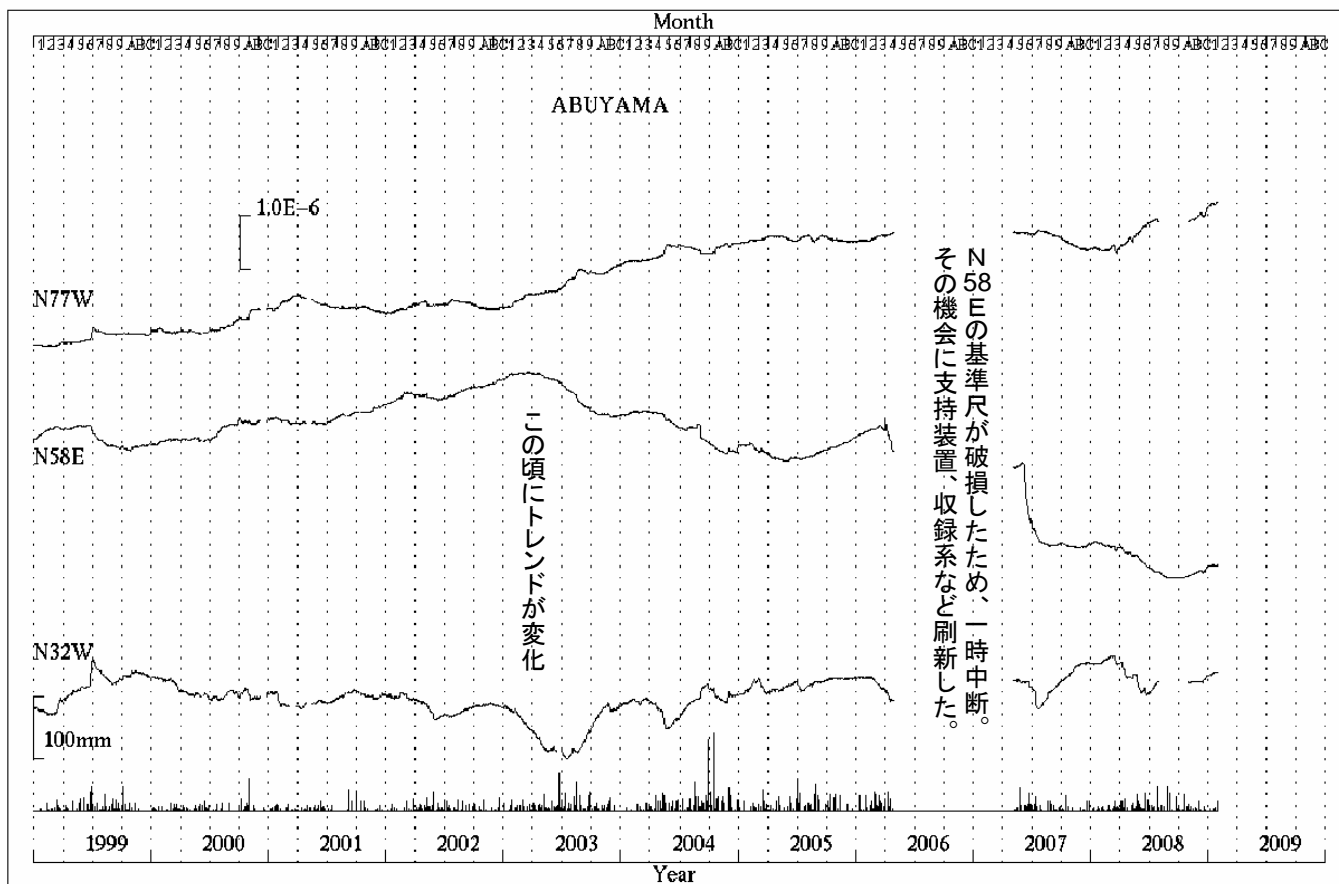
第4図 阿武山観測所における歪変化と日雨量（1999年1月～2009年2月）
