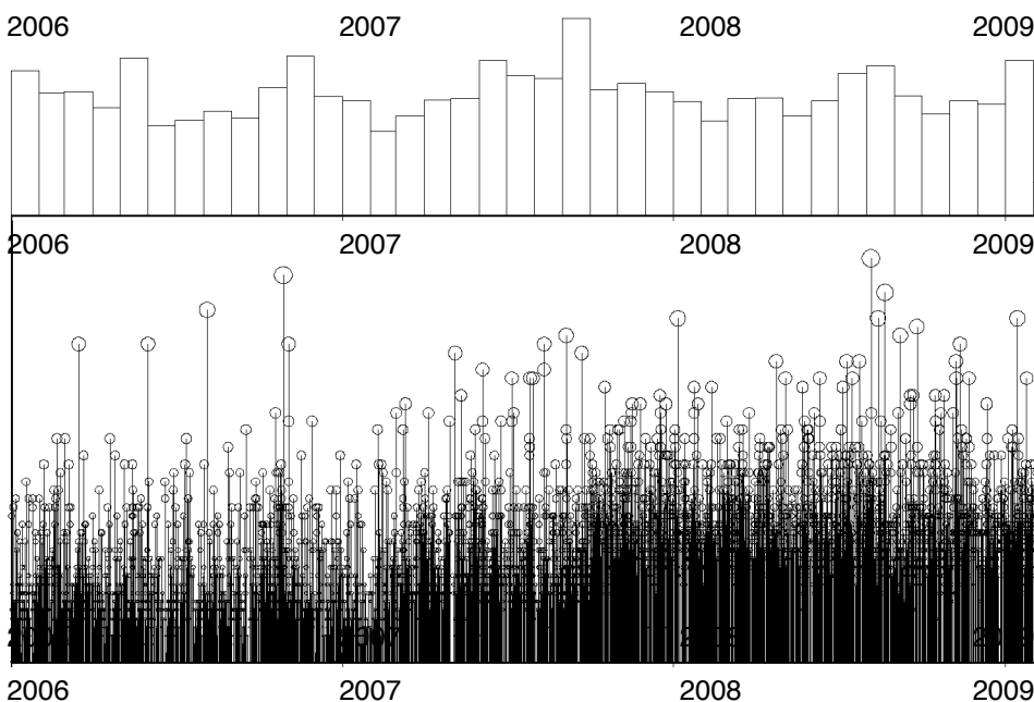
図3： (上) 2006年1月1日～2009年2月10日。30km以浅。京都大学防災研究所地震予知研究センターによる、図1の矩形範囲内の積算地震発生数。 赤い線はdeclusterしたカタログによる積算数。 (中) 同領域内における月別地震数。 (下) MT図。
