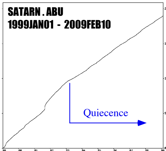
図2：1999年～2009年2月10日、図1の矩形内の積算発生数。
