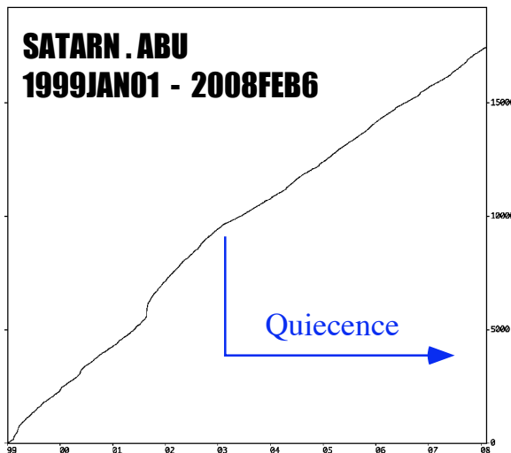
図2：1999年～2008年2月6日、図1の矩形内の積算発生数。
