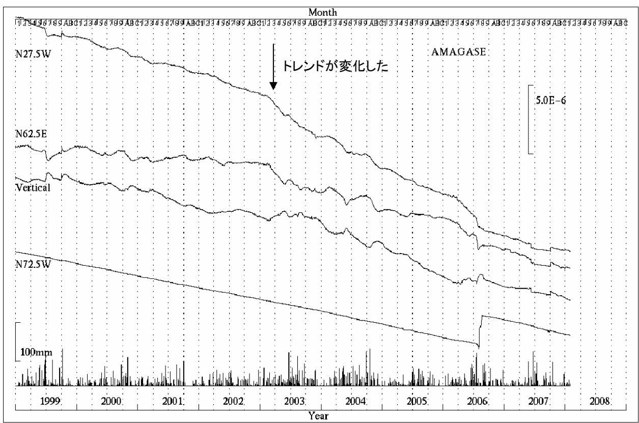
第1図 天ヶ瀬観測室における歪変化と日雨量（1999年1月～2008年1月）
